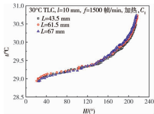
图 6 转静间隙对热色液晶标定的影响
