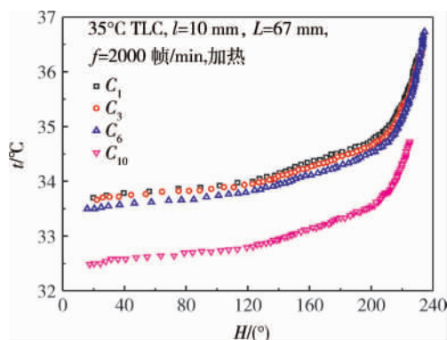
图8 加热老化对热色液晶标定的影响
