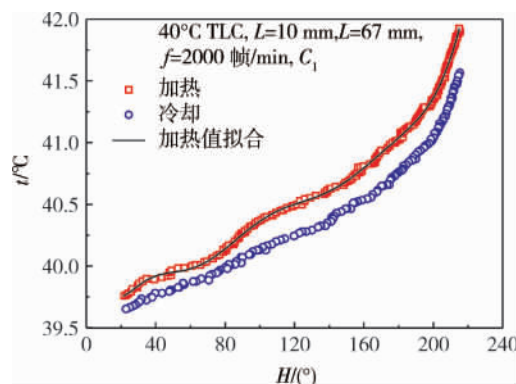
图9 滞后效应对热色液晶标定的影响
