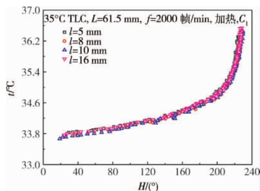
图 5 有机玻璃拍摄窗厚度对热色液晶标定的影响
