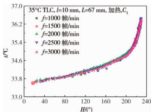
图7 频闪频率对热色液晶标定的影响
