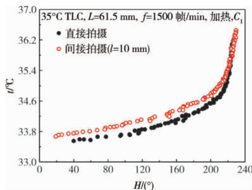
图 4 拍摄方式(直接和间接)对热色液晶标定的影响
