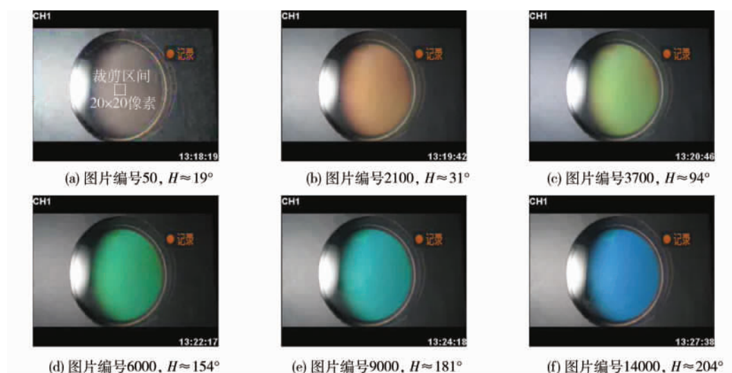
图3 典型热色液晶标定的颜色变化
